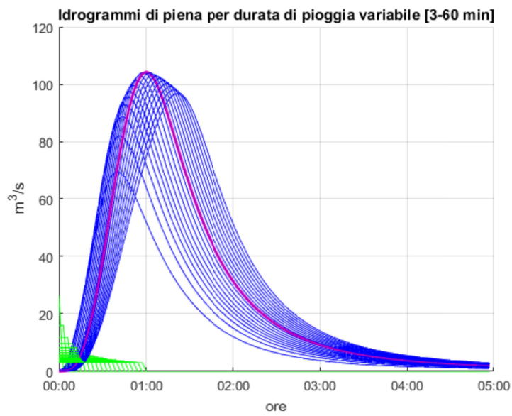
Figura A1 – Esempio dell'insieme degli idrogrammi calcolati per assegnato tempo di ritorno e diverse durate di pioggia. In rosso è evidenziato quello critico per massima portata al picco.
