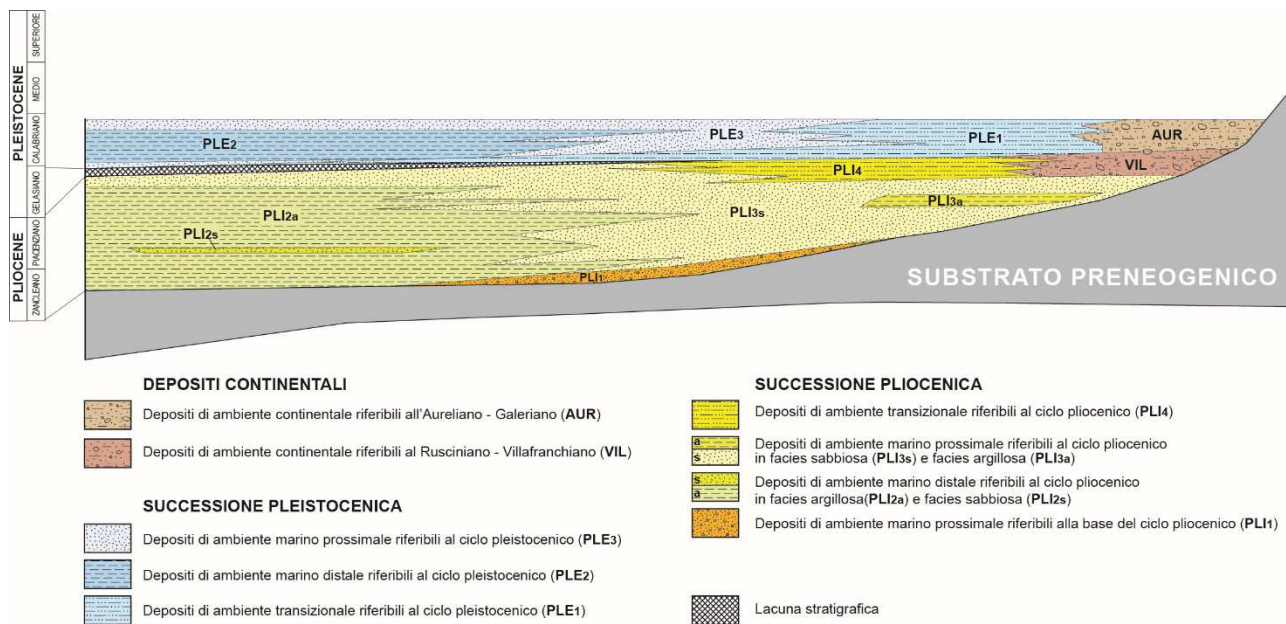
Fig. 3 – Rappresentazione schematica delle successioni stratigrafiche neogenico-quadernarie.
